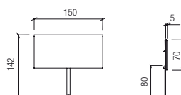
Vue de face Front view
