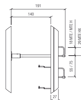
Détail Vue de côté Detail side view
