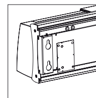
Fixation murale, pour montage sur placoplatre/brique Wall fixing for mounting onto plasterboard/brickwork
