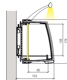
Vue de côté Side view
