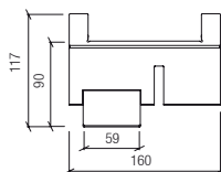
Vue de dessus Top view
