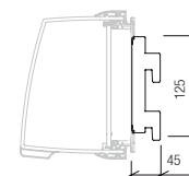
Vue de côté Side view
