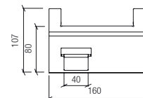
Vue de dessus Top view
