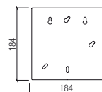
Vue arrière Back view
