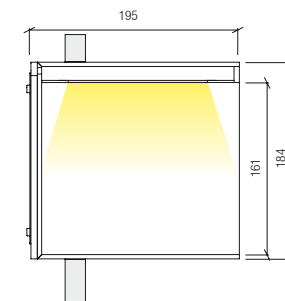
Vue de côté Side view
