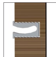
01. A Crémaillère LINEAR dans panneau bois LINEAR rail in wooden panel
