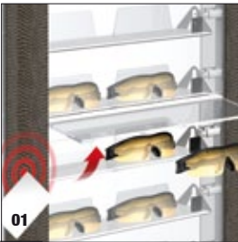
Trappe d'accès au produit Cover flap for output hopper
