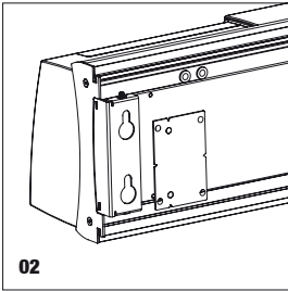
Fixation murale, par paire Wall fixing, one pair
