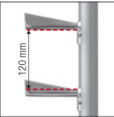
Beaucoup d'espace pour saisir confortablement les lunettes Plenty of space for taking out the spectacles comfortably
