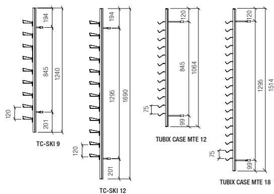
Vue de côté Side view
