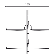
Détail. Vue de face Detail front view
