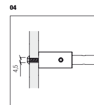
Montage sur acrylique Mounting onto acrylic glass
