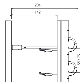
Détail. Vue de côté Detail side view
